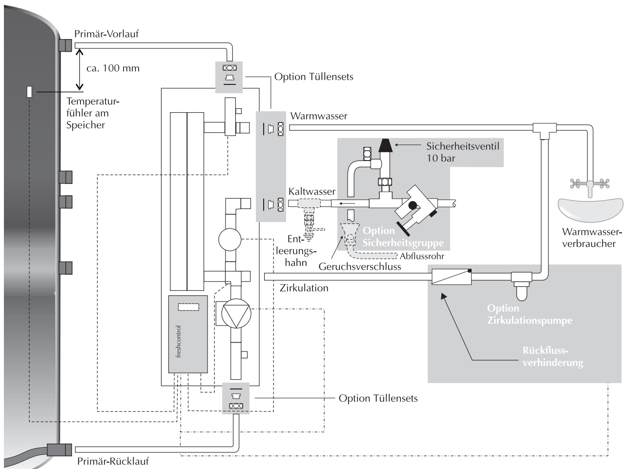
Bild 3 RATIOfresh Anschlussplan nach DIN 1988
