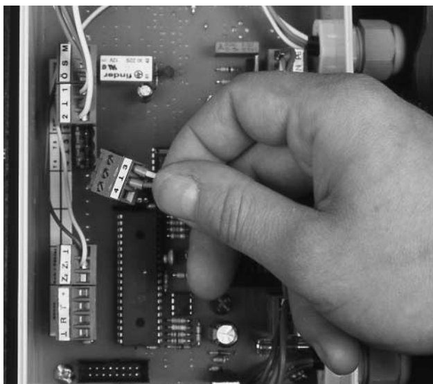
Bild 14 Option "Weitere Temperaturfühler anschließen": Regler spannungsfrei schalten (nur Fachpersonal), nach Klemmenplan (Bild 22) anschließen.
