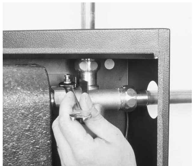
Bild 15 Pufferspeicher befüllen, Primärkreislauf entlüften. Dazu Netzstecker einstecken und Primärkreispumpe auf Dauer-Ein (BAW1 = EIN) schalten.
