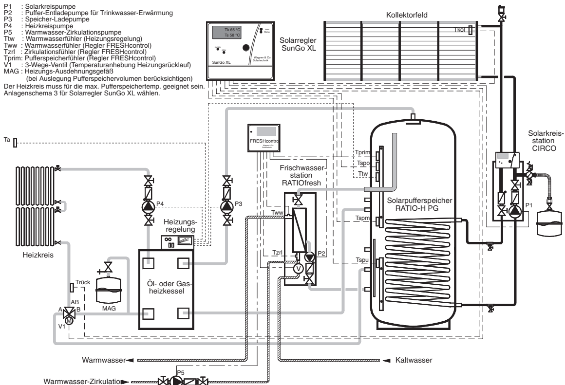
Bild 27 Solaranlage für Warmwasserbereitung und Heizungsunterstützung. Systemlösung in Verbindung mit Öl- oder Gaskessel, Pufferspeicher RATIO-H PG und Frischwasserstation RATIOfresh. Die Warmwasserbereitung erfolgt im elektronisch geregelten Durchflusserfahren. Der Regler der Frischwasserstation FRESHcontrol sorgt für eine konstante Entnahmetemperatur und besonders niedrige Rücklauftemperaturen für den Pufferspeicher. Solarenergie für die Raumheizung wird über eine Anhebung der Rücklauftemperatur des Heizkreises genutzt, wenn im Pufferspeicher eine ausreichende Temperatur vorliegt.
