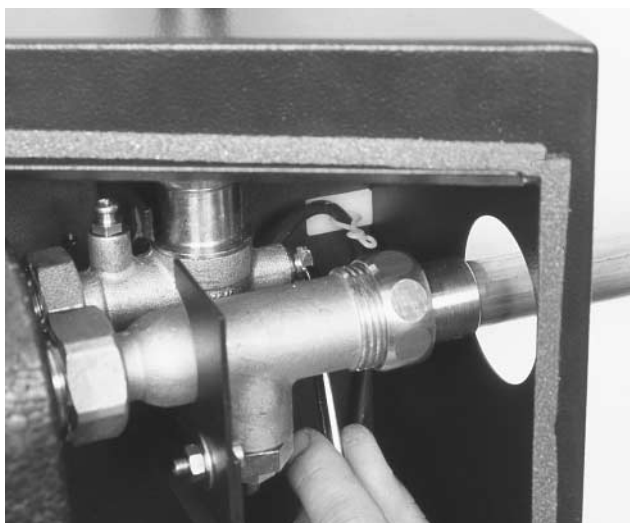
Bild 25 Absperrhahn im Primärkreis-Vorlauf und Pumpenschieber zum Absperrn des Primärkreises schließen.
