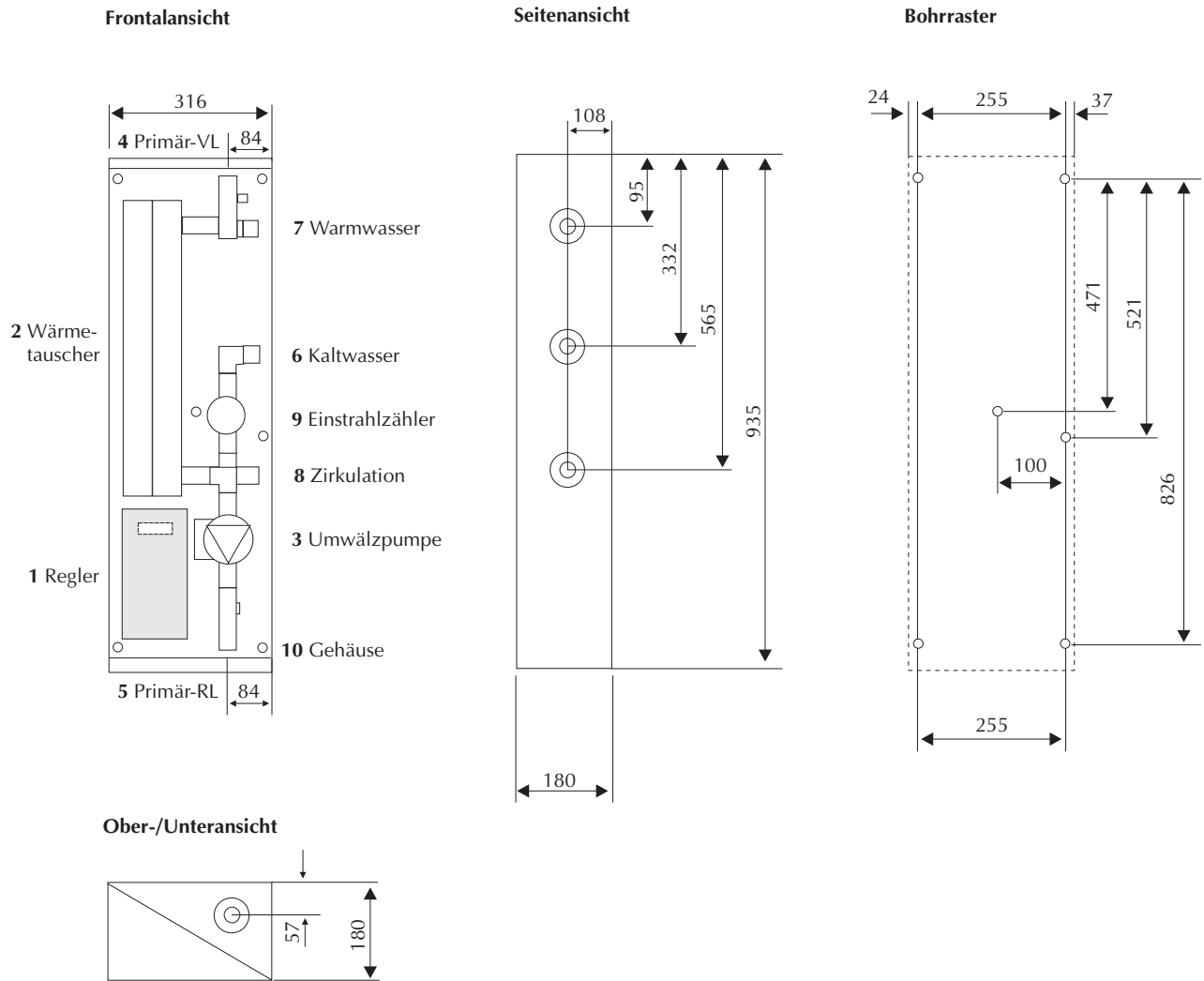
Bild 2 RATIOfresh Frischwasserstation im Schnitt mit Maßen und Bohrraster 1 FRESHcontrol - adaptive Microprozessorregelung zur Warmwasser- u. Zirkulationsregelung. Display 1 x 16 Zeichen, Folientastatur mit 3 Tasten und 4 LED, 2 Leistungsausgänge; inkl. 1 Volumenstromzähler, 3 Temperaturfühler und 2 Tauchhülsen aus verchromtem Messing, 2 Plattenwärmeübertrager aus Edelstahl, kupfergelötet. Flachdichtende Anschlüsse G 1" (AG) - schneller Ausbau zu Wartungsarbeiten. Übertragerleistung: 61 kW bzw. 98 kW. Speziell geprägte Plattenstruktur zur Vermeidung von Kalkablagerungen. Komplett mit EPP-Schalendämmung (expandiertes Polypropylen), 3 Umwälzpumpe im Primärücklauf. Besonders energiesparende Ausführung. Wartungsfreundlich durch flachdichtende Einbindung, 4 Primärvorlauf- Anschluss G 1" (AG, flachdichtend) aus Messing, mit Absperrhahn und Entlüftung, 5 Primärücklauf- Anschluss G 1" (AG, flachdichtend) aus Messing, mit Pumpenabsperrierschieber inkl. Rückflussverhinderer, 6 Kaltwasserzulauf- Anschluss G 1" (AG, flachdichtend) aus Messing, 7 Warmwasserablauf- Anschluss G 1" (AG, flachdichtend) aus Messing mit Temperaturfühler in Tauchhülse, 8 Zirkulationsrücklauf- Anschlussmöglichkeit G 1/2" (IG), mit Stopfen verschlossen. Temperaturfühler in Tauchhülse, 9 Einstrahlzähler- Messing, verchromt, Anschlüsse 3/4" (AG), flachdichtend. QN: 2,5 m³/h, 18 Imp./l, 10 Gehäuse - aus zweifarbig pulverbeschichtetem Stahlblech, Gehäusedeckel abnehmbar. Unterteil mit Schlüsselbohrungen zur Wandmontage.
