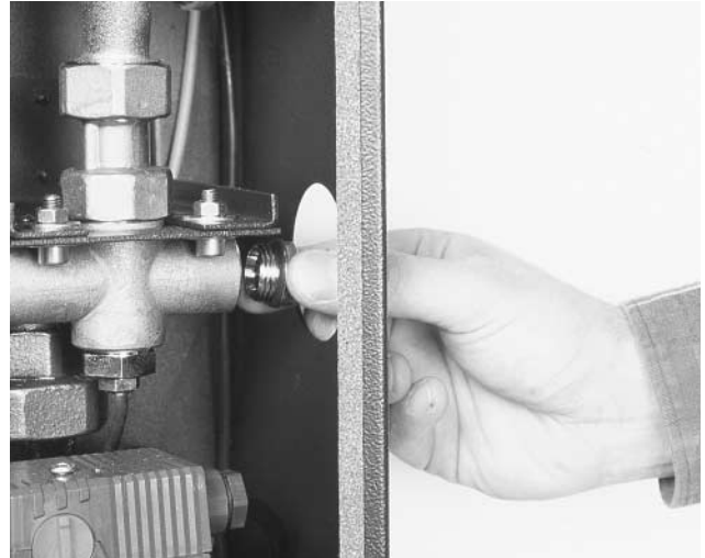
Bild 11 Option Zirkulation: An Zirkulations-RL-Anschluss Stopfen 1/2" entfernen ...
