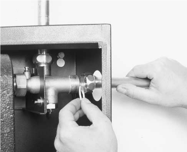
Bild 10 Warmwasser anschließen. Gut dämmen. Flachdichtungen nicht vergessen !
