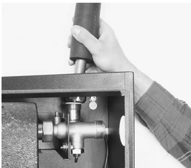
Bild 6 Primär-VL-Leitung aus heißstem Speicherbereich zur Ratiofresh-Frischwasserstation führen und anschließen. Bei ansteigender Leitungsführung Entlüfter einbauen.
