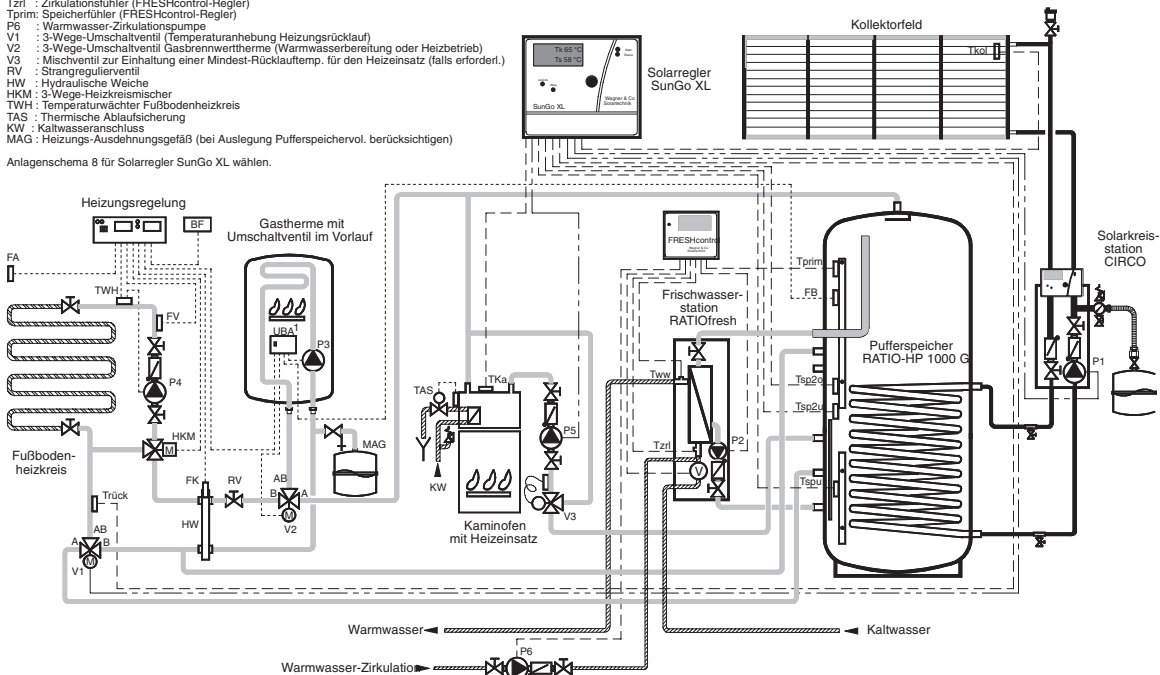
Bild 28 Solaranlage für Warmwasserbereitung und Heizungsunterstützung. Systemlösung mit Gasterme, Kaminofen mit Heizeinsatz, RATIO-Pufferspeicher, Frischwasserstation RATIOfresh und einem Fußbodenheizkreis. Die Warmwasserbereitung erfolgt im elektronisch geregelten Durchflusserfahren. Der Kaminofen heizt den oberen Pufferspeicherbereich auf, Solarenergie kann den gesamten Pufferspeicher erwärmen. Bei ausreichenden Temperaturen im Speicher, wird über das Umschaltventil V1 der Heizungsrücklauf durch den Speicher geführt und Pufferspeicherenergie für die Raumheizung genutzt. Der Solarregler steuert zusätzlich die Pufferbeladung durch den Kaminofeneinsatz.
