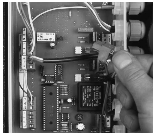
Bild 13 Regler spannungsfrei schalten (nur Fachpersonal), bauseitige Zirkulationspumpe nach Klemmenplan (Bild 22) anschließen.
